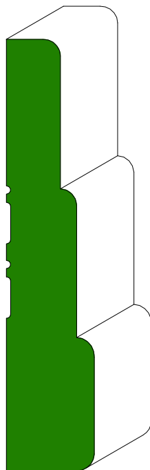
LRM 683 5/8 x 3-1/4 WF - Random
